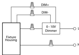
0 - 10V Wiring
