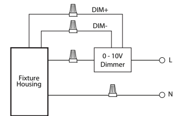
0 - 10V Wiring
