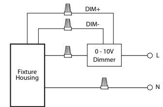
0 - 10V Wiring
