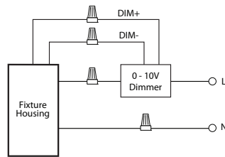
0 - 10V Wiring
