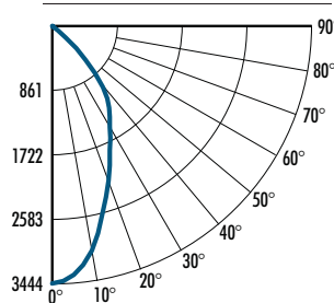
CANDELA TABULATION
