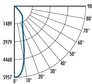
CANDELA TABULATION
