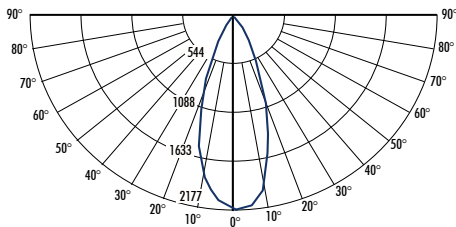
CANDELA TABULATION
